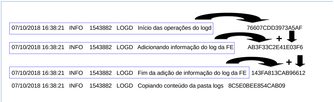
Figura 2 – Exemplo de composição da autenticação do log.
